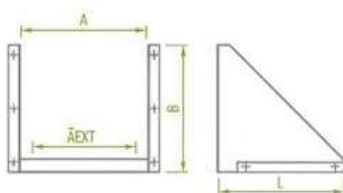
Soporte mural
