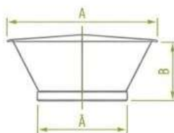
Caperuza plana
